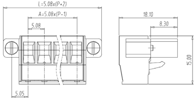
■ 图示(Pic. shown) : TLPSW-300V-1067-06P-G12S
